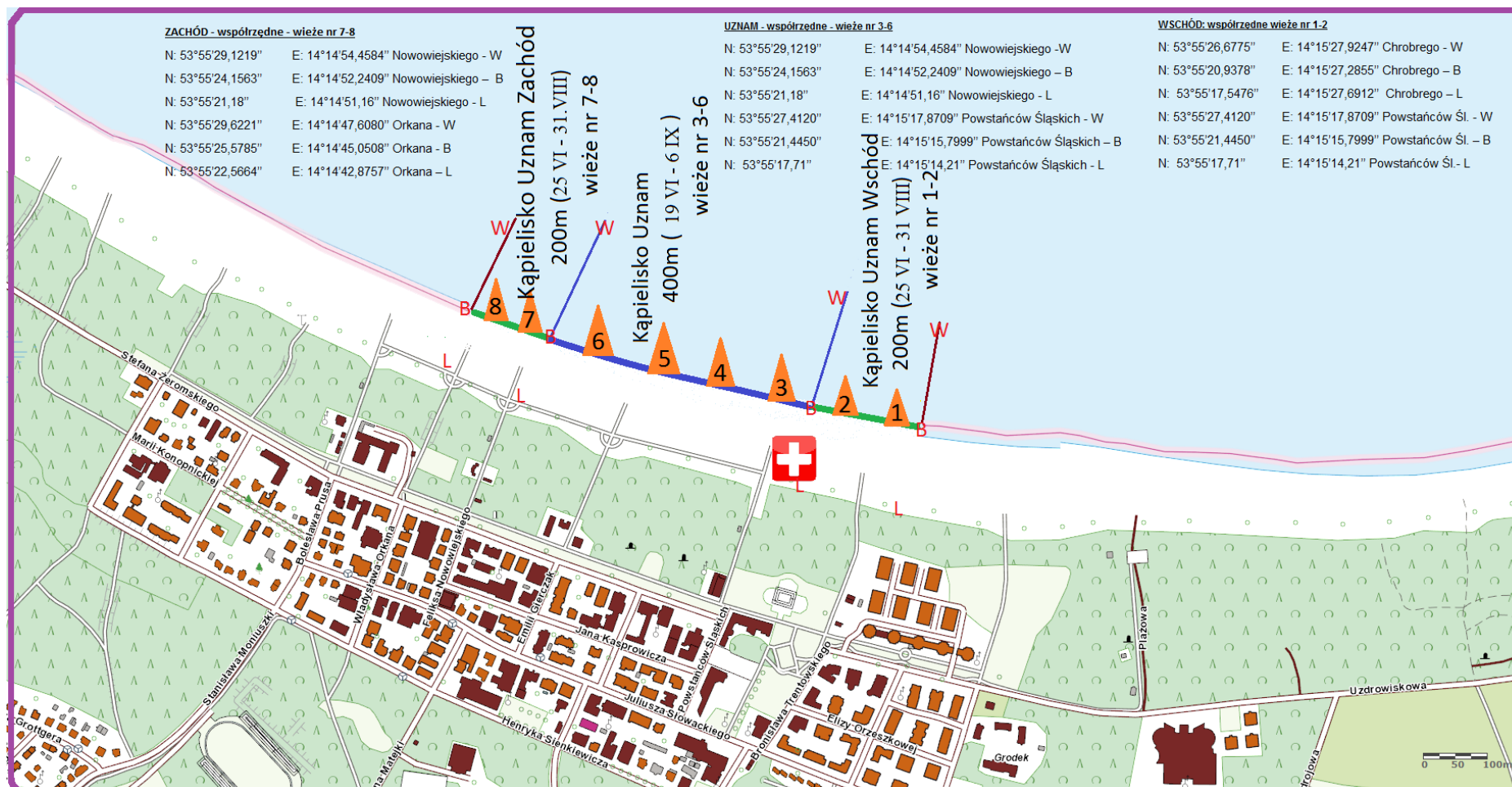
Szkie 1 Obszar zabezpieczenia Kąpiełisk Morskich Świnoujście Zachód w sezonie 2020
